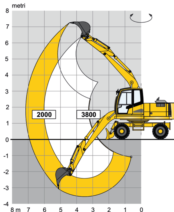
DIAGRAMMA DELLE PORTATE (daN) SUI 360° DI ROTAZIONE CONTINUA
